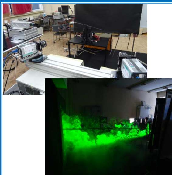
СПЕЦИАЛИЗИРАНА СИСТЕМА ЗА ИЗМЕРВАНЕ НА ФЛУИДНИ ПОТОЦИ
