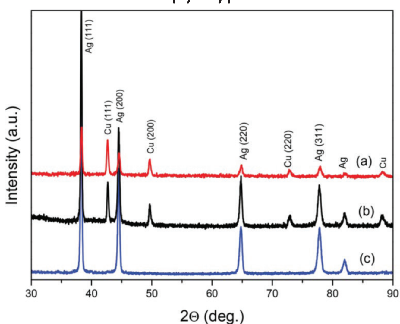
Рентгеноструктурен анализ
