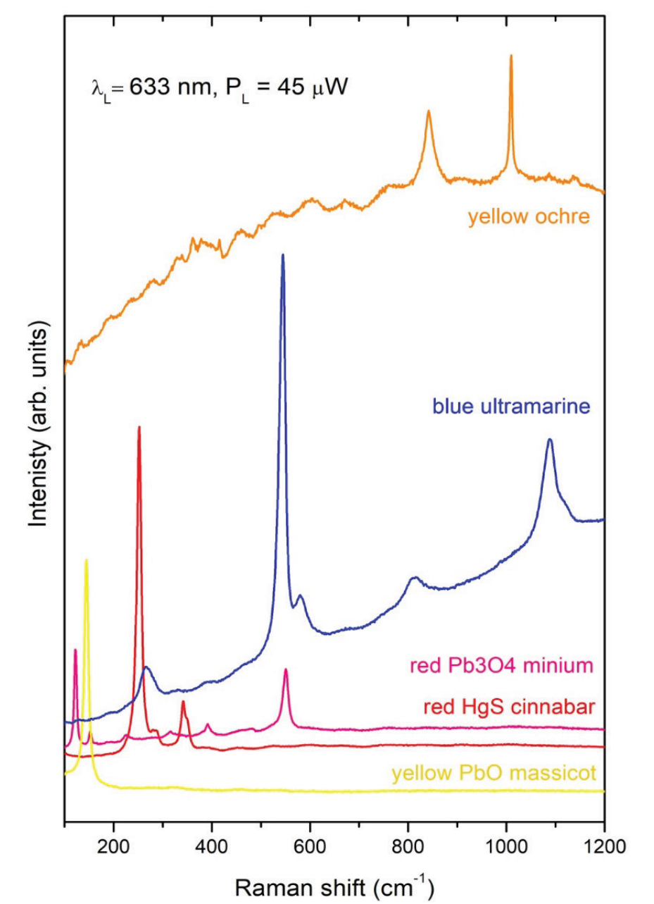
Раманова спектроскопия
